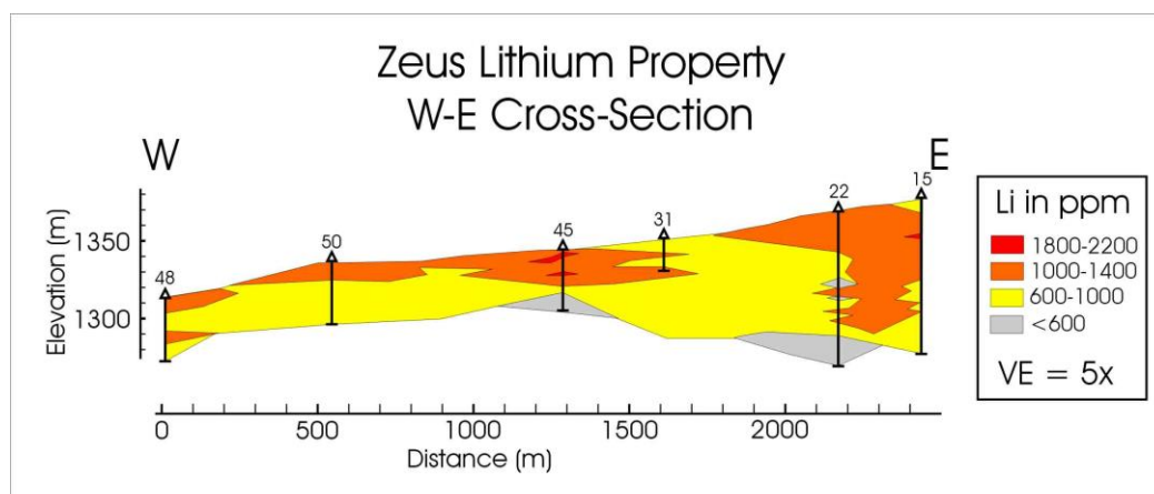
Abbildung 2. West-Ost-Querschnitt durch die bekannte Mineralisierung in Lithium-Tonsteinen der Esmeralda-Formation, kategorisiert nach Gehalt. Beachten Sie, dass das Gelände nach Osten ansteigt und der Gehalt und die Mächtigkeit in dieser Richtung am höchsten sind.
