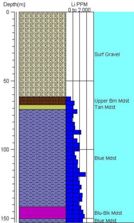
Abbildung 1a) Abstraktionsprofil von CVZ-67 mit den verschiedenen Schlammeinsteintypen, die ab der Oberfläche bis zu einer Tiefe von 502 Fuß (153 m) vorgefunden wurden
